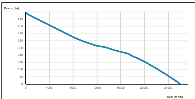
CAXIDIK 800-5-30
