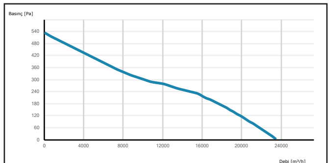
BAXI 800-5-30
