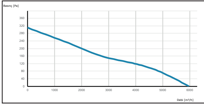
HAXI 500-5-25
