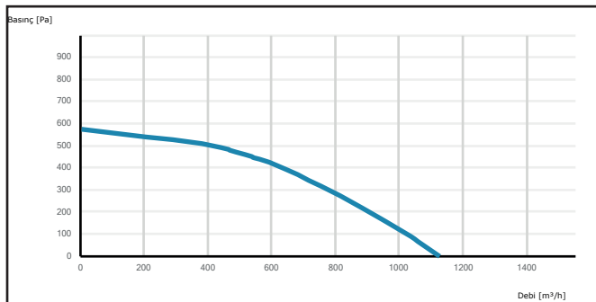
RAD 250
