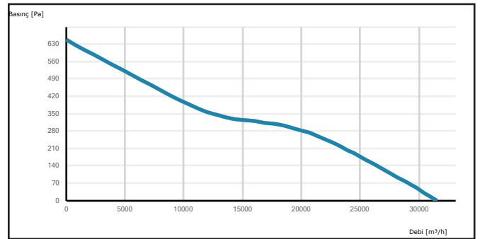
AXI 800-5-35
