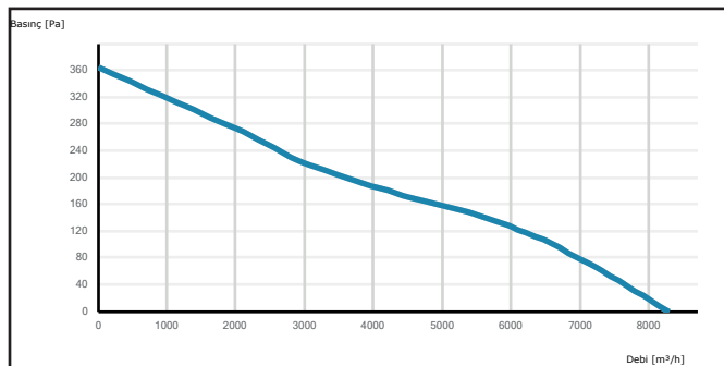
CTAXI 560-5-25
