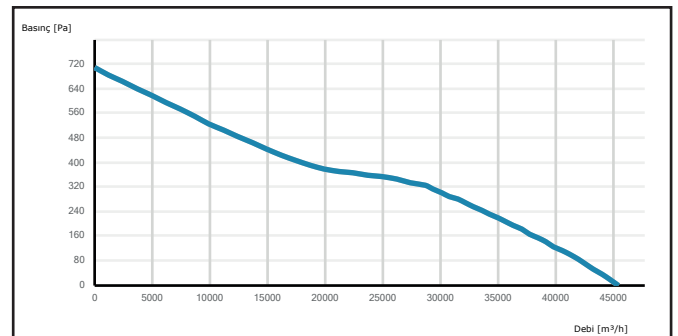
DAXI 900-5-40
