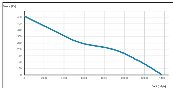
PAXI 630-5-30
