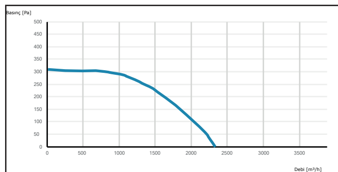
DRAD 355
