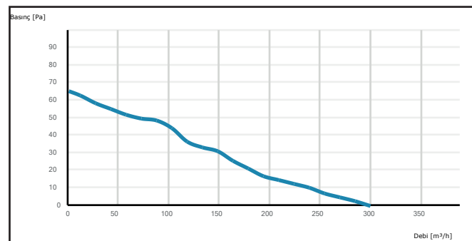
YUF 160
