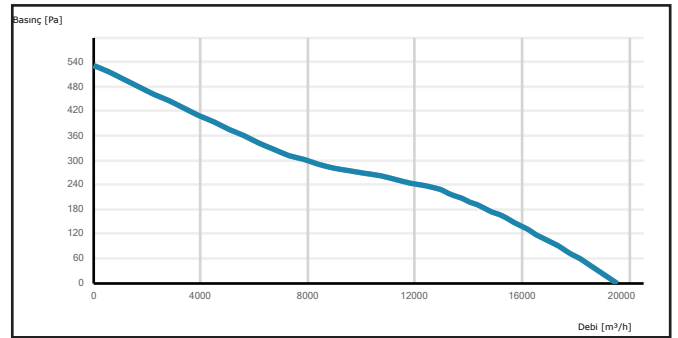
AXI 710-5-30
