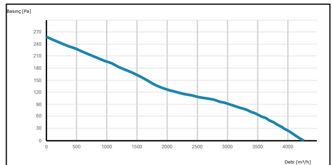
CAXIDIK 450-5-25
