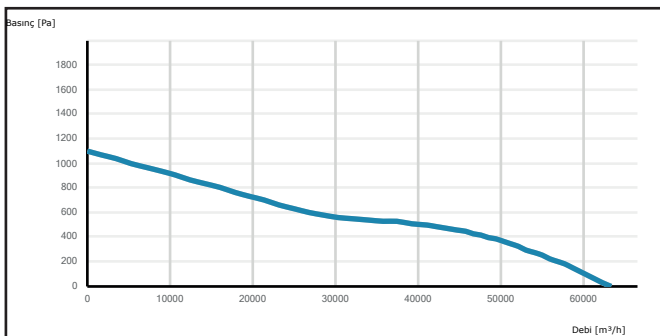
DAXI 1000-8-40
