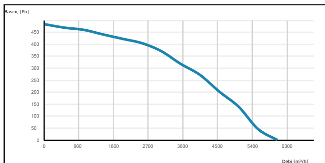
IGK 50
