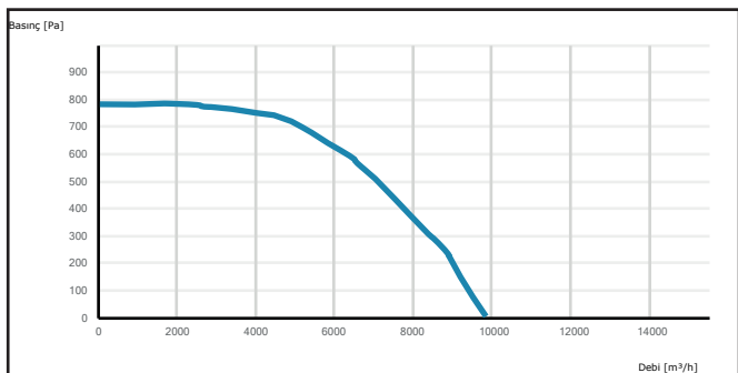
DREC 560
