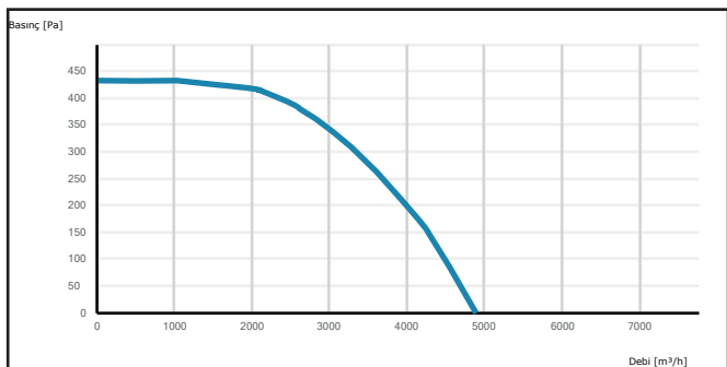
CRAD 450
