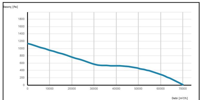
DAXI 1000-8-45
