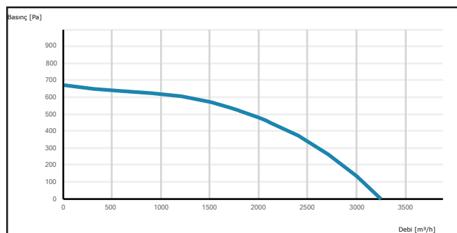
EC-CRAD 315
