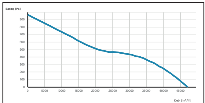
DAXI 900-8-40
