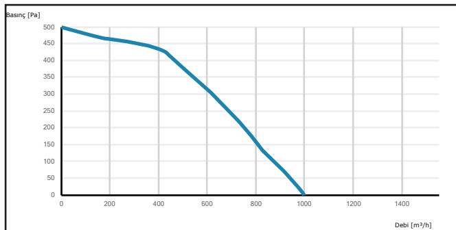
RAD 200
