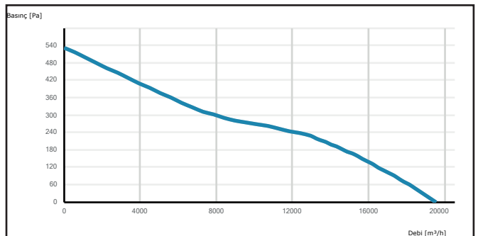
AXIP 710-5-30
