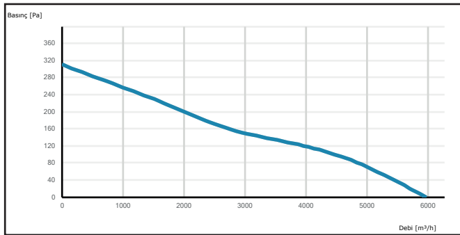
CAXIDIK 500-5-25
