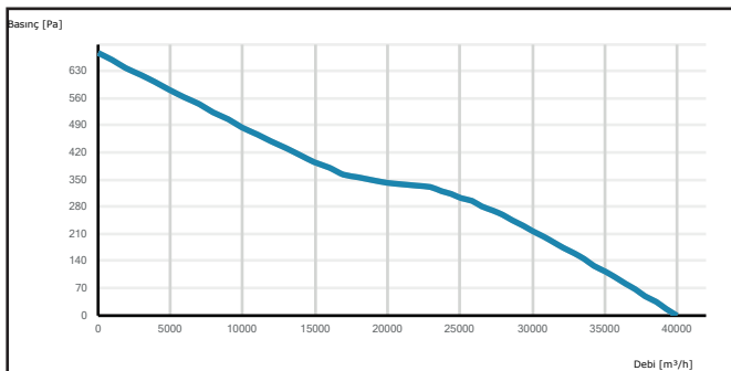
HAXI 900-5-35
