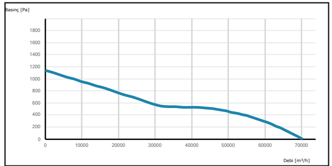
AXI 1000-8-45
