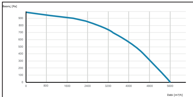
EC-CRAD 355
