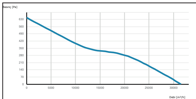
PAXI 800-5-35
