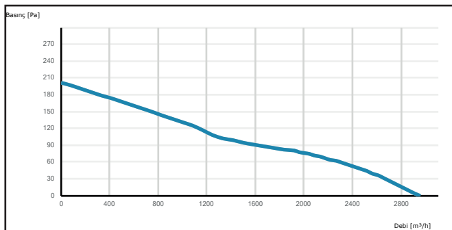
HAXI 400-5-25
