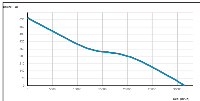
CTAXI 800-5-35
