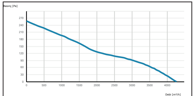
AXIP 450-5-25
