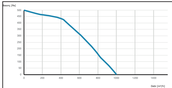
CRADIK 225
