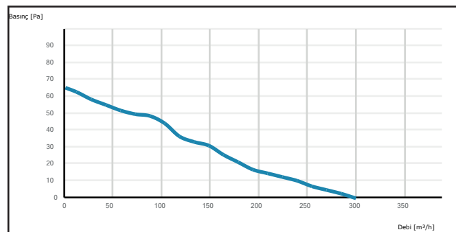
YUF 150
