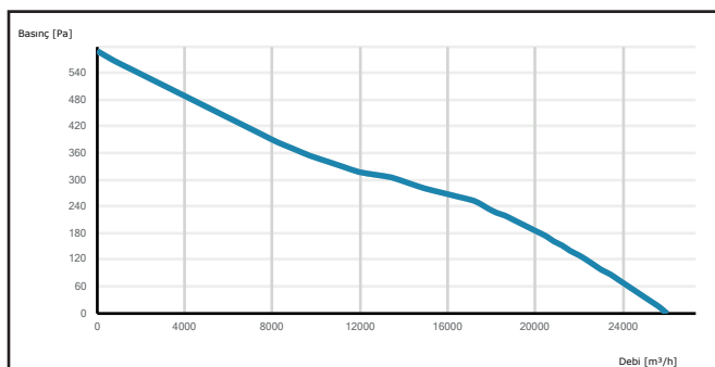
CTAXI 800-5-30
