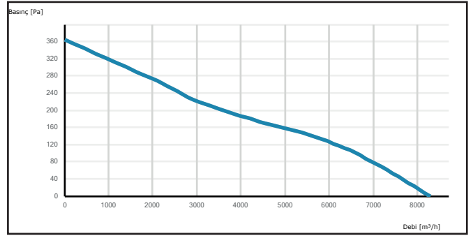
DAXI 560-5-25
