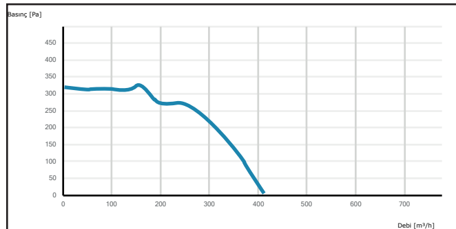
RAD 125
