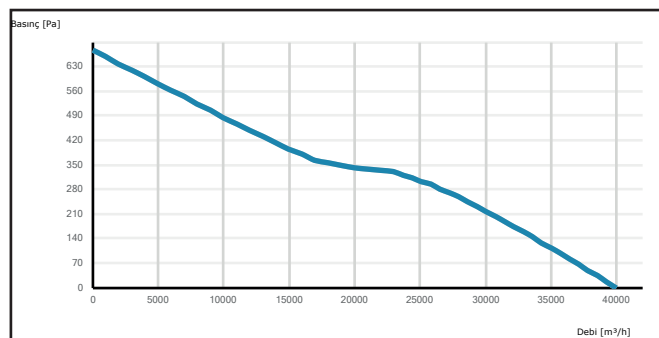
PAXI 900-5-35
