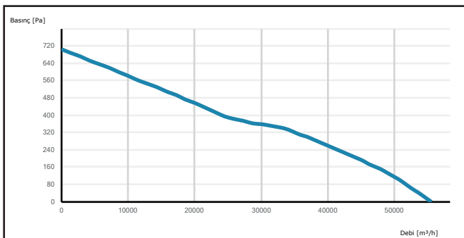
CTAXI 1000-5-40
