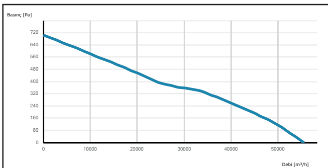
AXIP 1000-5-40
