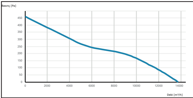
AXI 630-5-30
