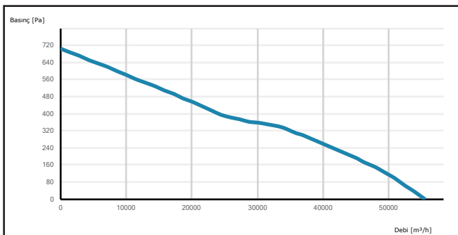
CTAXI 1000-5-40
