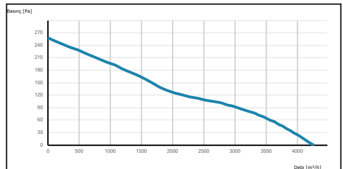
AXI 450-5-25
