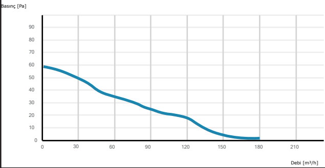
SEF 125
