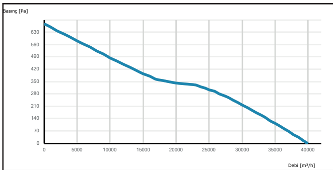
AXI 900-5-35
