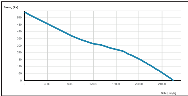
AXI 800-5-30
